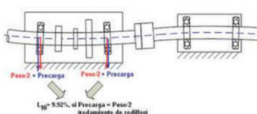
MAQUINAS DESALINEADAS: Fuerzas sobre cada rodamiento = Peso rotor/2 + Precarga,F
